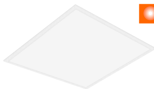
PANEL LD 60X60 33W 84 3630LM Cód.: 317902
